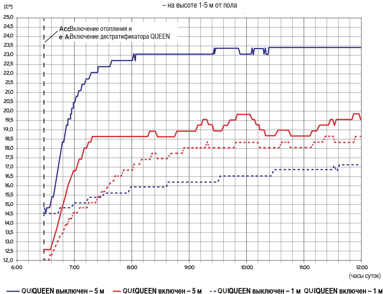
СОПОСТАВЛЕНИЕ ТЕМПЕРАТУР В ПОМЕЩЕНИИ ПРИ ВКЛЮЧЕННОМ И ВЫКЛЮЧЕННОМ ДЕСТРАТИФИКАТОРЕ — на высоте 1-5 м от пола
